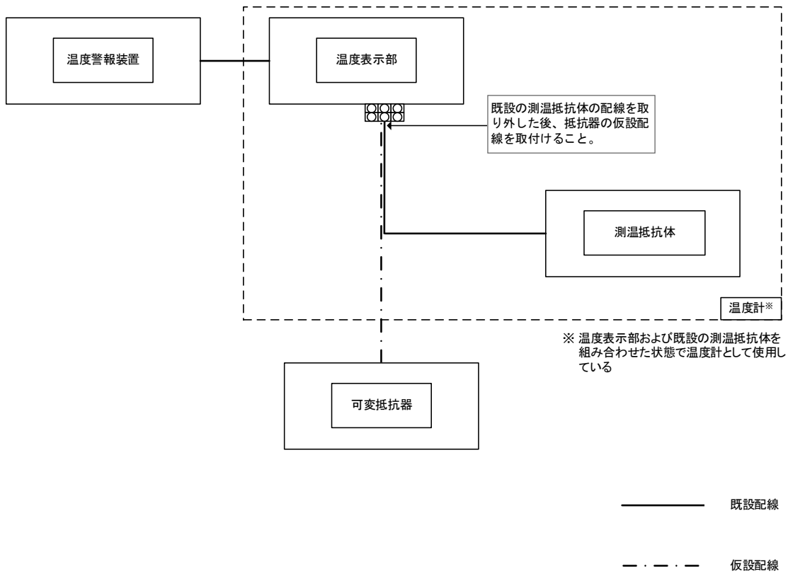
図一 2 温度計の接続図
